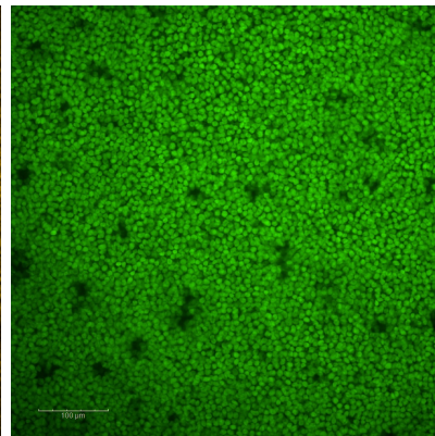
Otx2
