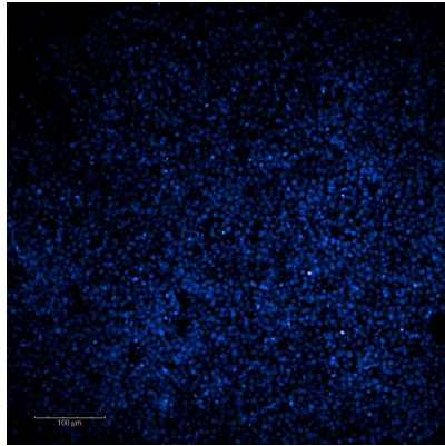
DAPI
