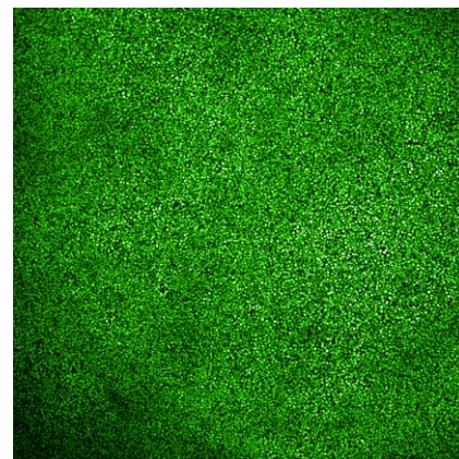
Otx2
